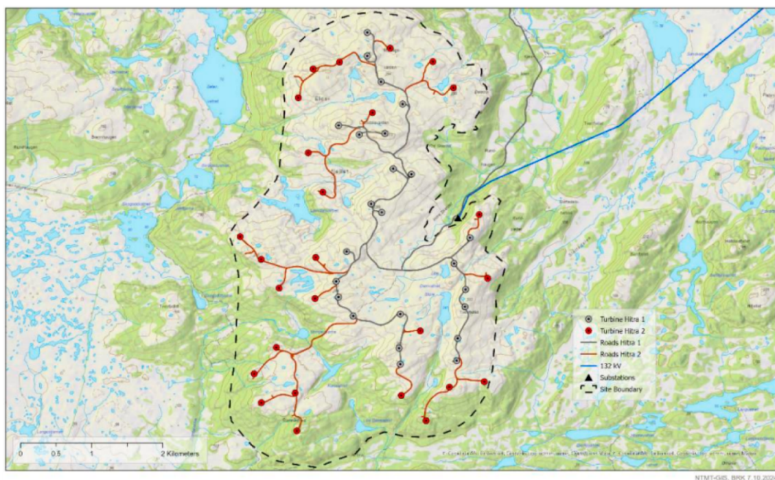
Figur 5 Kart som viser dagens Hitra 1 og Hitra 2 vindkraftverk. Turbinene til Hitra 1 i grått og turbinene til Hitra 2 i rødt.
