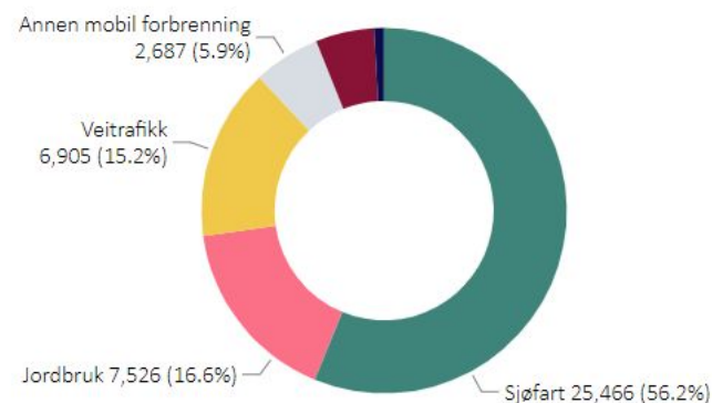
Utslipp (tonn CO 2 -ekvivalenter) per sektor i Hitra i 2021
