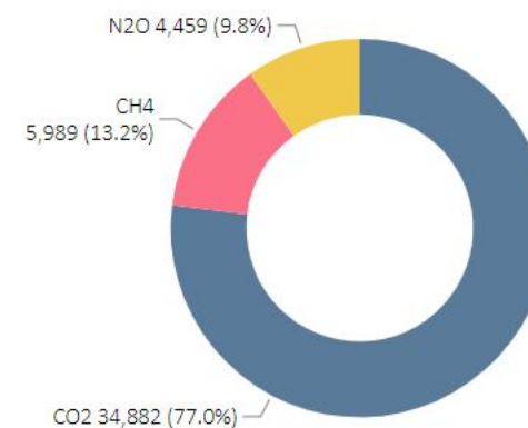
Utslipp (tonn CO 2 -ekvivalenter) i Hitra i 2021 per klimagass
